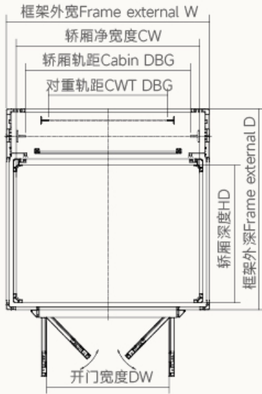
平台梯
