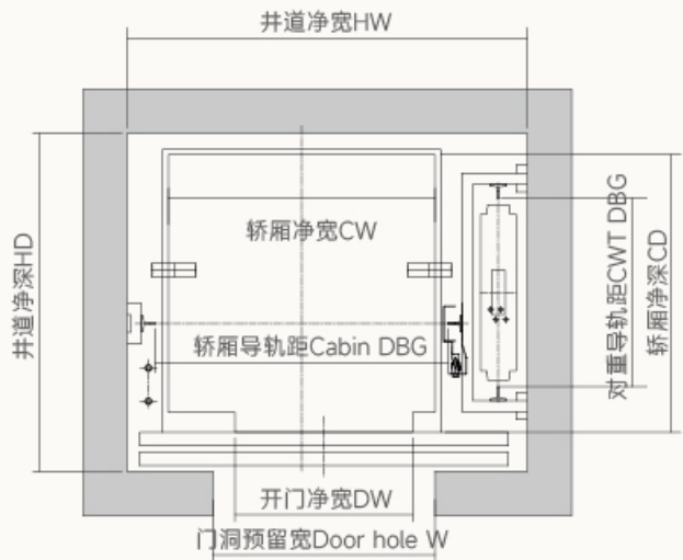
钢丝绳侧置轿底轮
